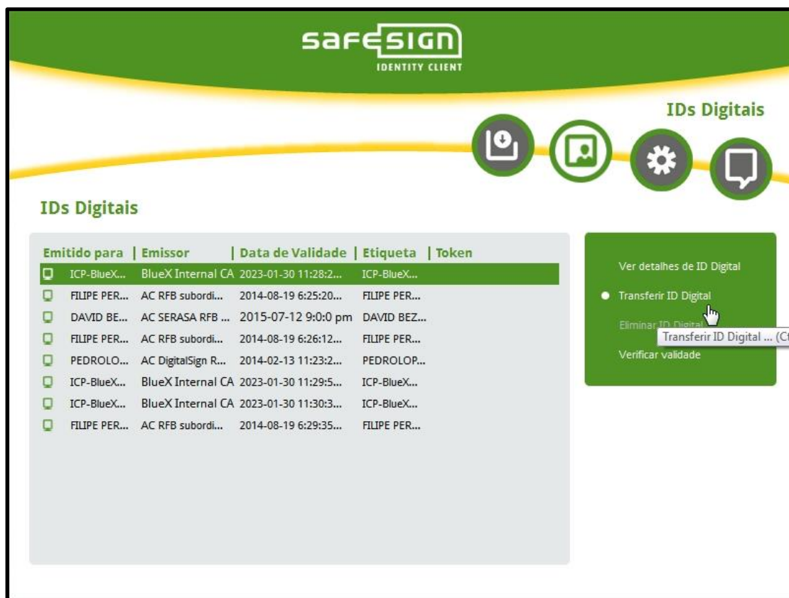
Figura 26: IDs Digitais: Transferir ID para o token
