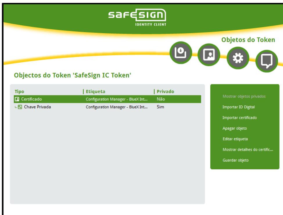
Figura 95: Objetos PKCS#11: Todos os objetos
